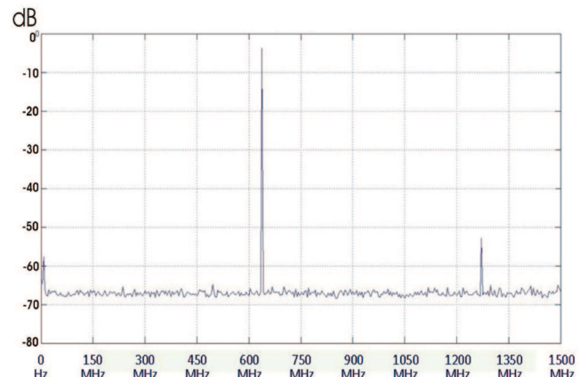
DAC SFDR
